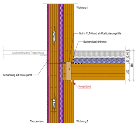
Konstruktion Treppenhauswand
