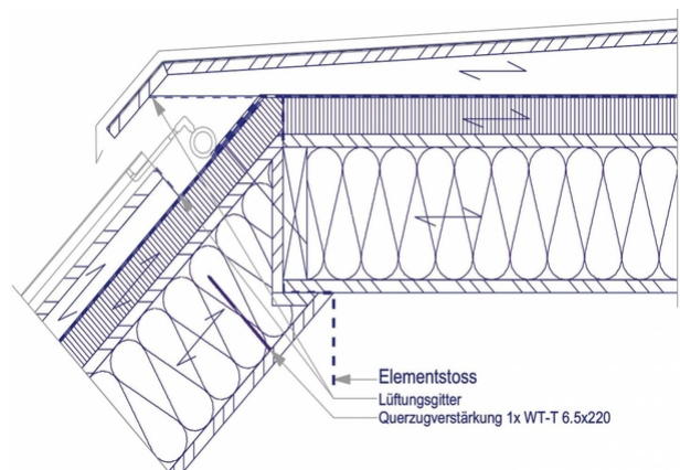
Detail Wand-Deckenstoss
