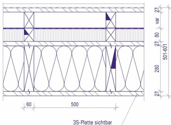
Detail Deckenaufbau
