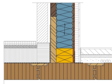
Anschluss Geschosdecke - Terrasse an Aussenwand
