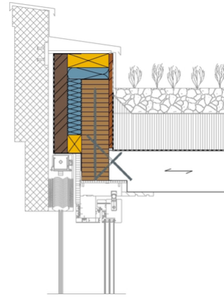
Anschluss Flachdach an bestehende Aussenwand
